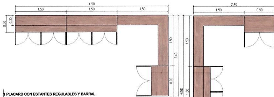
VISTA A
